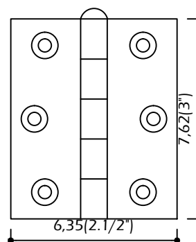
DOBRADIÇA 3"x 2.1/2"
