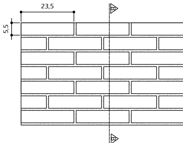
ELEVAÇÃO ESCALA 1/10
