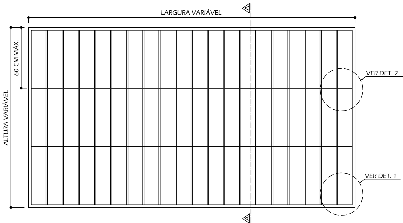
ELEVAÇÃO ESCALA 1/20
