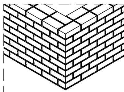
AMARRAÇÃO CONVENCIONAL DE ALVENARIA DE CANTO SEM ESCALA
