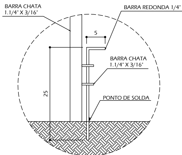
DETALHE 2 - FERROLHO ESCALA 1/5
