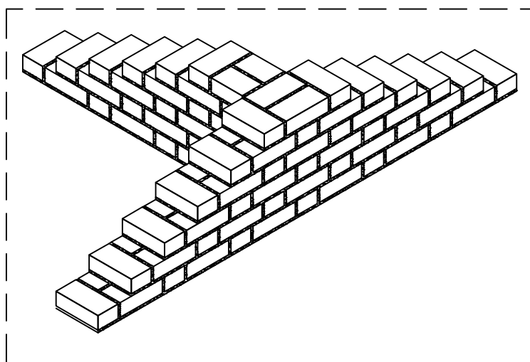
AMARRAÇÃO INGLESA DE ALVENARIA INTERMEDIÁRIA
