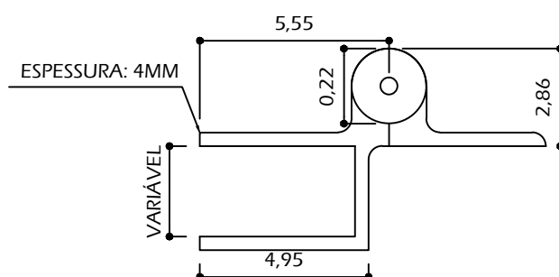
DETALHE DOBRADIÇA ESCALA 1/2
