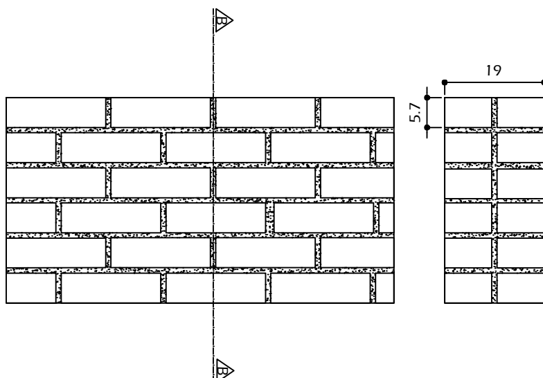
AMARRAÇÃO CONVENCIONAL ELEVÇÃO ESCALA 1/10
