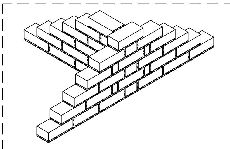
AMARRAÇÃO DE ALVENARIA INTERMEDIÁRIA SEM ESCALA
