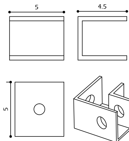
SUPORE PARA DUAS PEDRAS DE CANTO
