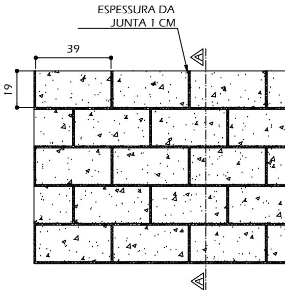
ELEVACÃO
