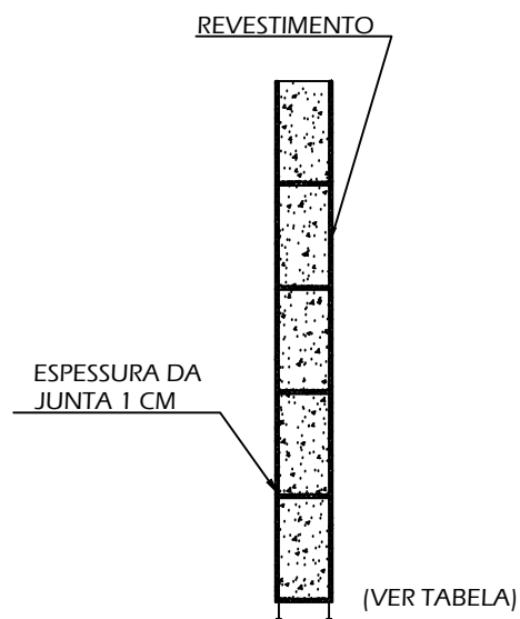
CORTE A-A ESCALA 1/25
