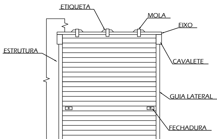
ELEVAÇÃO ESCALA 1/50
