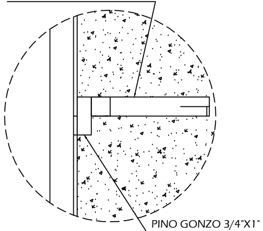
DETALHE 3
