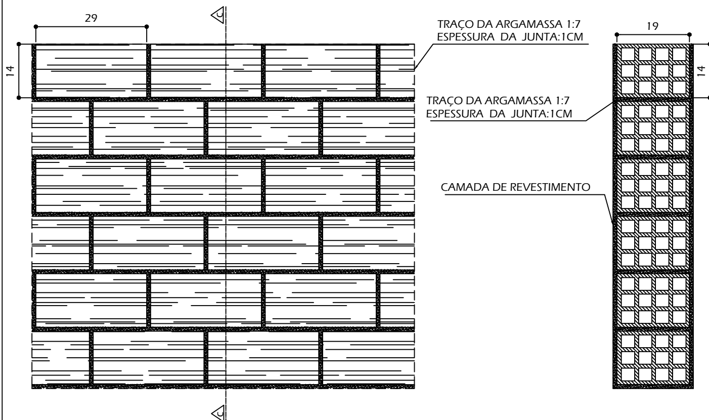
CORTE C-C ESCALA 1/10
