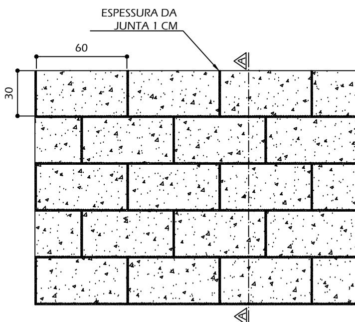
ELEVAÇÃO ESCALA 1/25
