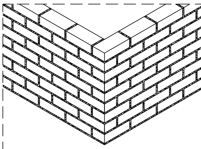
AMARRAÇÃO DE ALVENARIA DE CANTO SEM ESCALA
