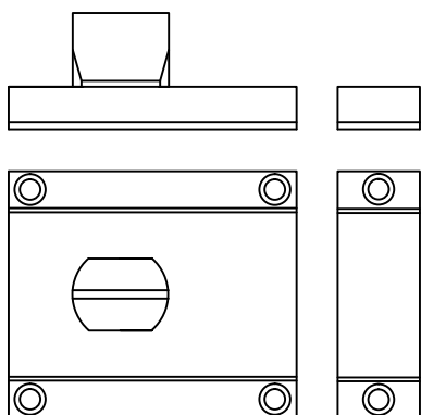
VISTA POSTERIOR TARJETA LIVRE/OCUPADO
