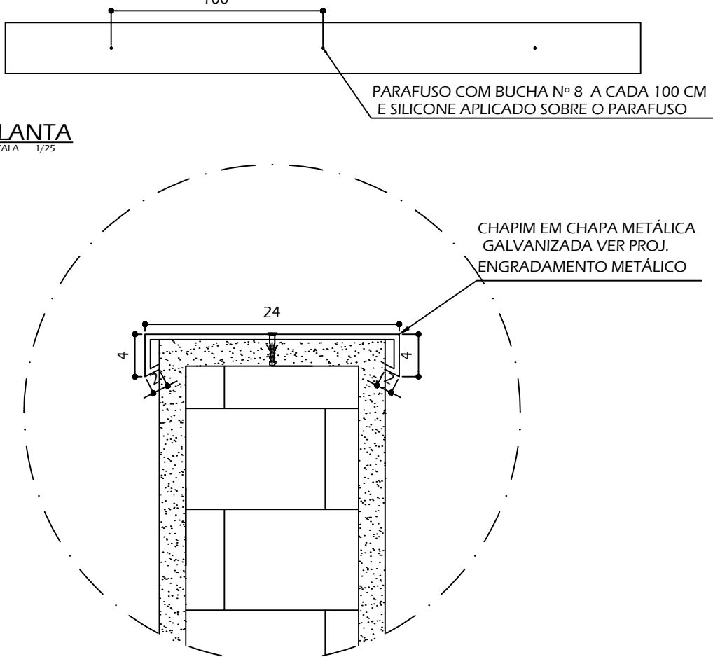
DETALHE 1 ESCALA 1/5
