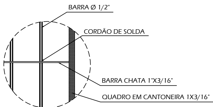
DETALHE 1 ESCALA 1/10
