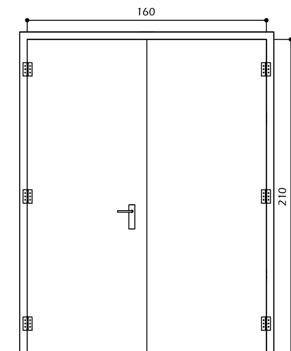
VISTA FRONTAL - PORTA 2 FOLHAS
