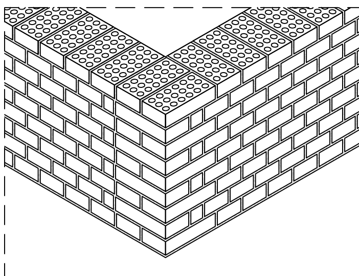
AMARRAÇÃO DE ALVENARIA DE CANTO SEM ESCALA
