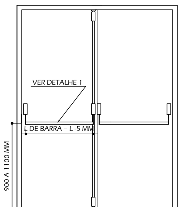
VISTA POSTERIOR - PORTA 2 FOLHAS
