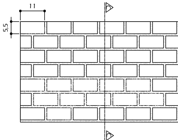
ELEVACÃO ESCALA 1/10
