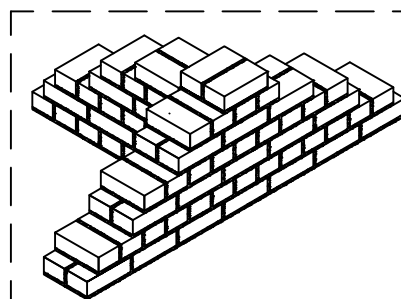
AMARRAÇÃO FRANCESA DE ALVENARIA INTERMEDIÁRIA SEM ESCALA
