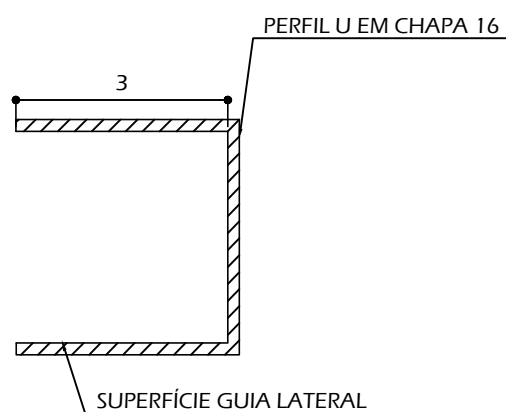
DETALHE GUIA LATERAL ESCALA 1/1
