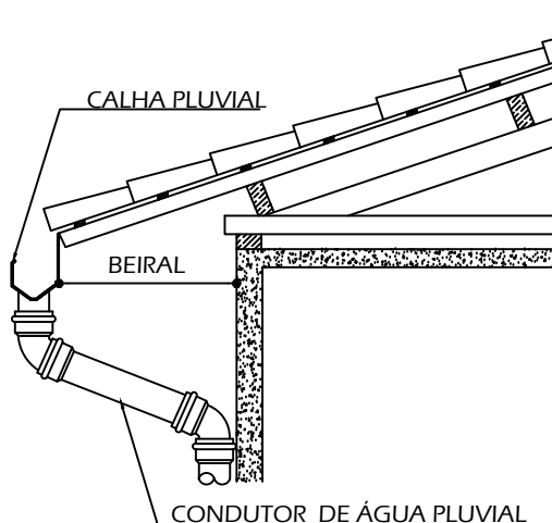
DETALHE 1 - LIGAÇÃO EM TELHADO COM BEIRAL SEM ESCALA
