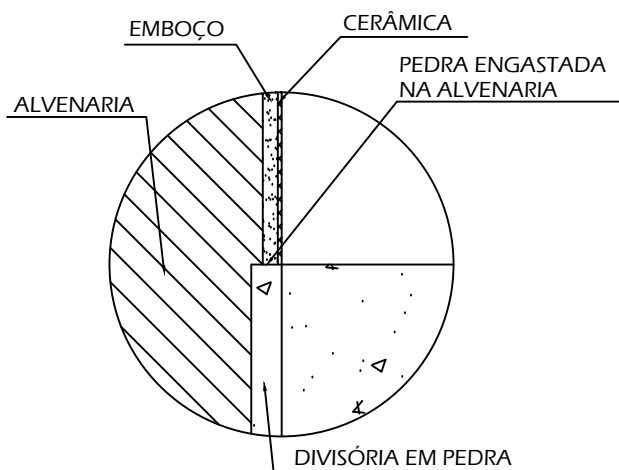
DETALHE 3 ESCALA 1/5
