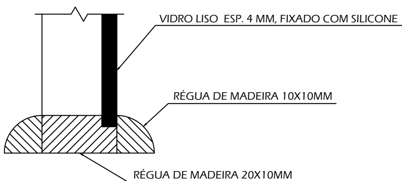
DETALHE 1
