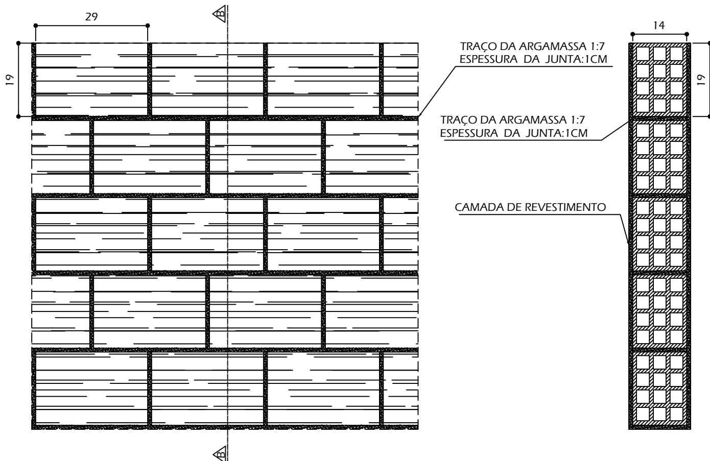
CORTE B-B
