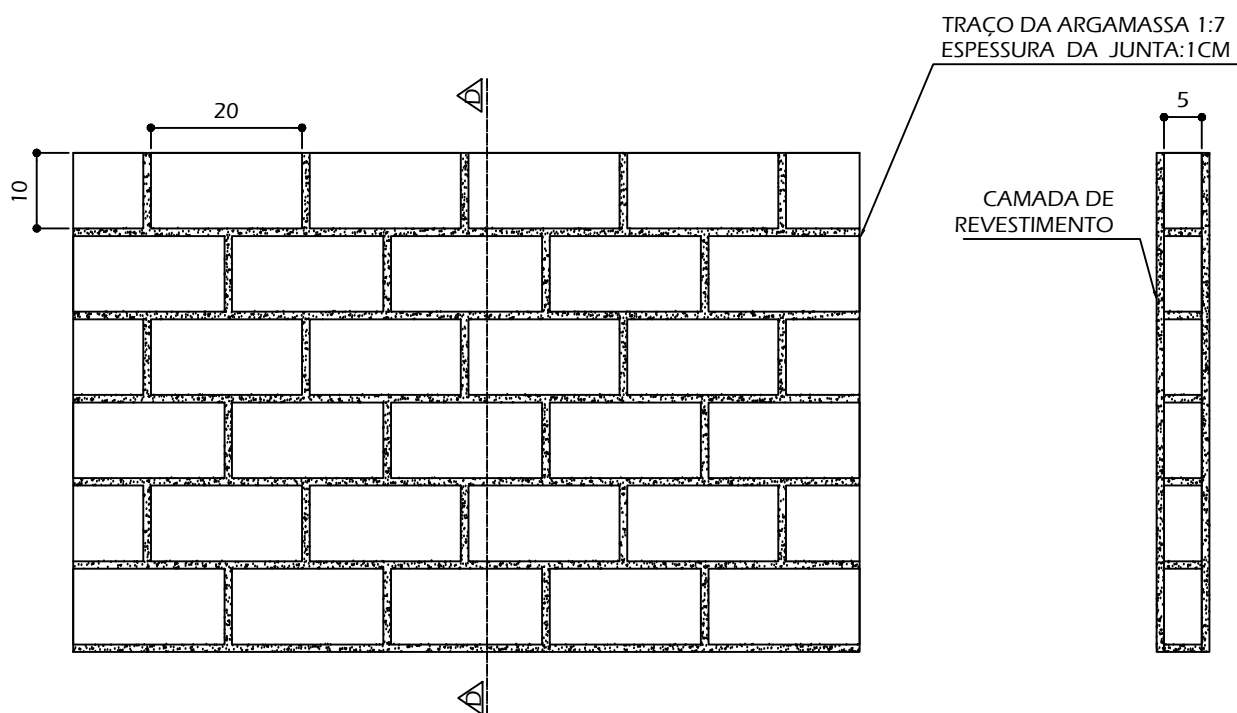
CORTE D-D ESCALA 1/10
