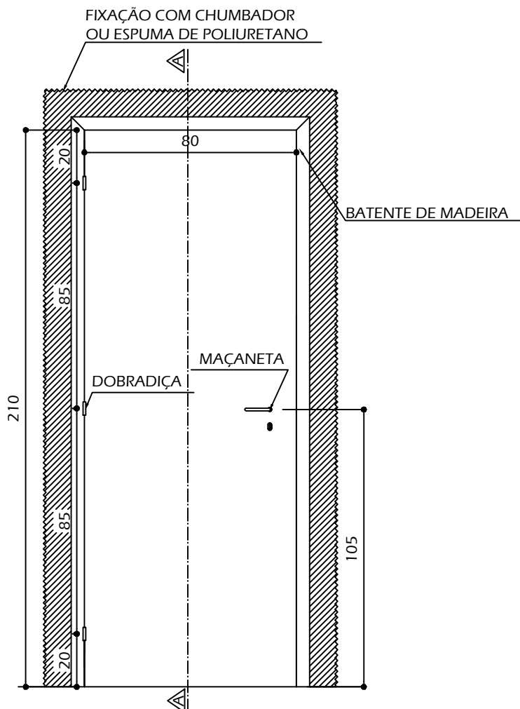
ELEVACÃO FRONTAL
