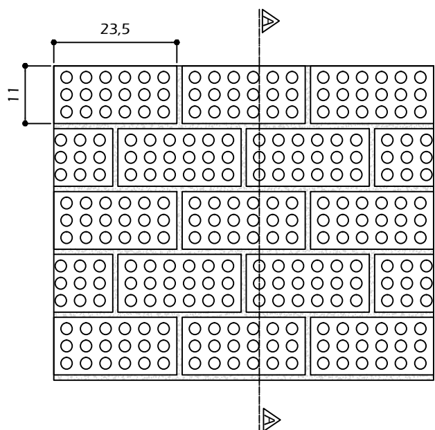
ELEVAÇÃO ESCALA 1/10
