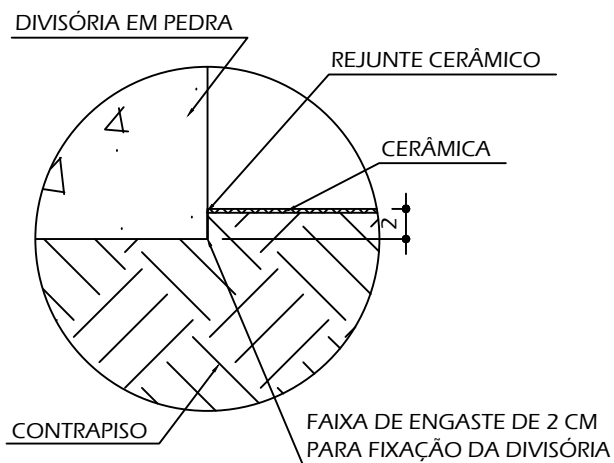
DETALHE 4 ESCALA 1/5
