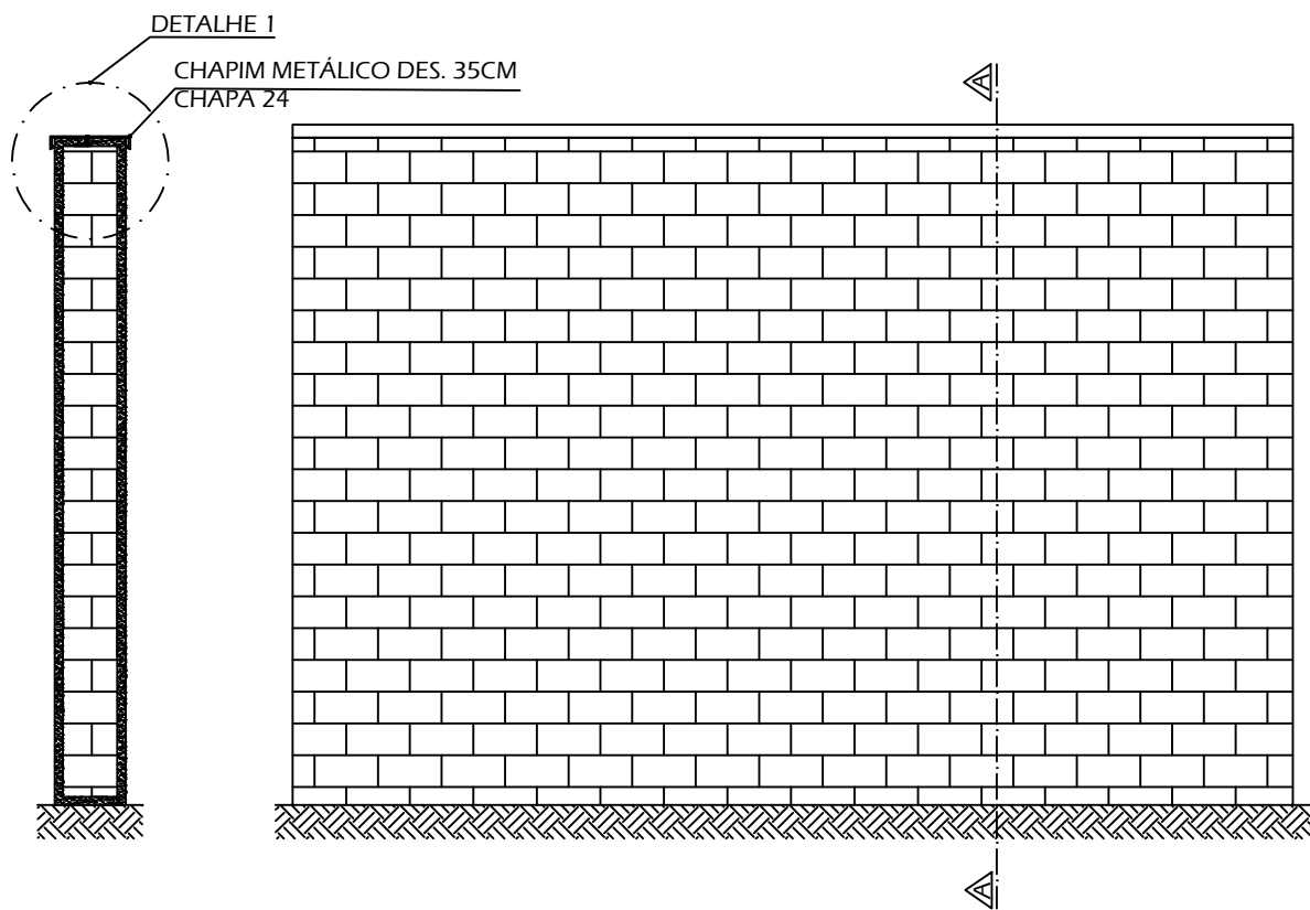
ELEVACÃO ESCALA 1/25 100
