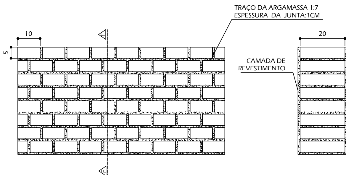
CORTE F-F ESCALA 1/10
