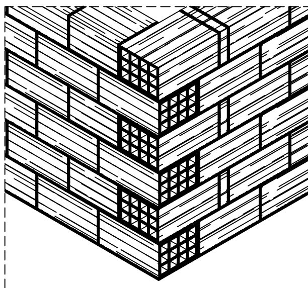
PERSPECTIVA DE AMARRAÇÃO DAS ALVENARIAS SEM ESCALA
