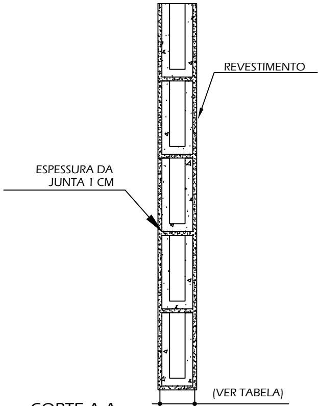
CORTE A-A
