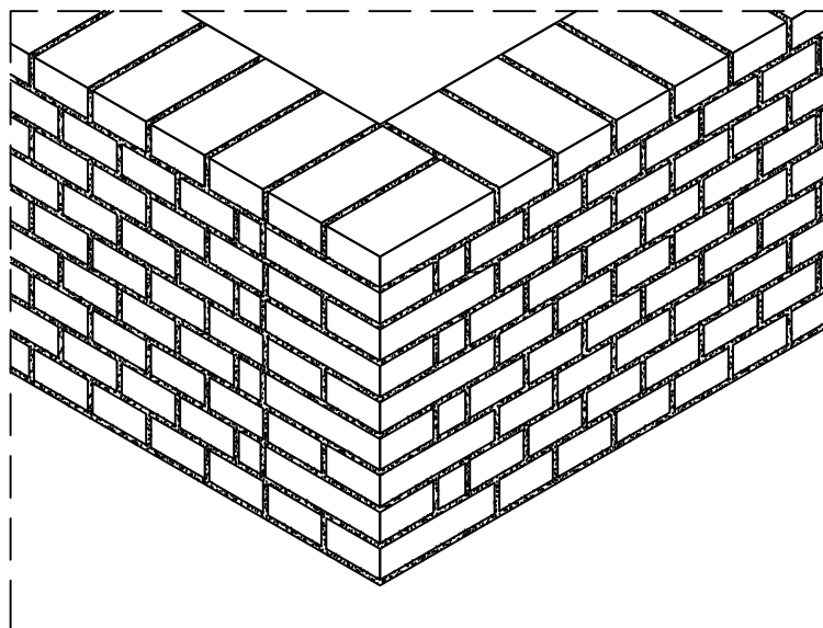
PERSPECTIVA DE AMARRAÇÃO DAS ALVENARIAS SEM ESCALA
