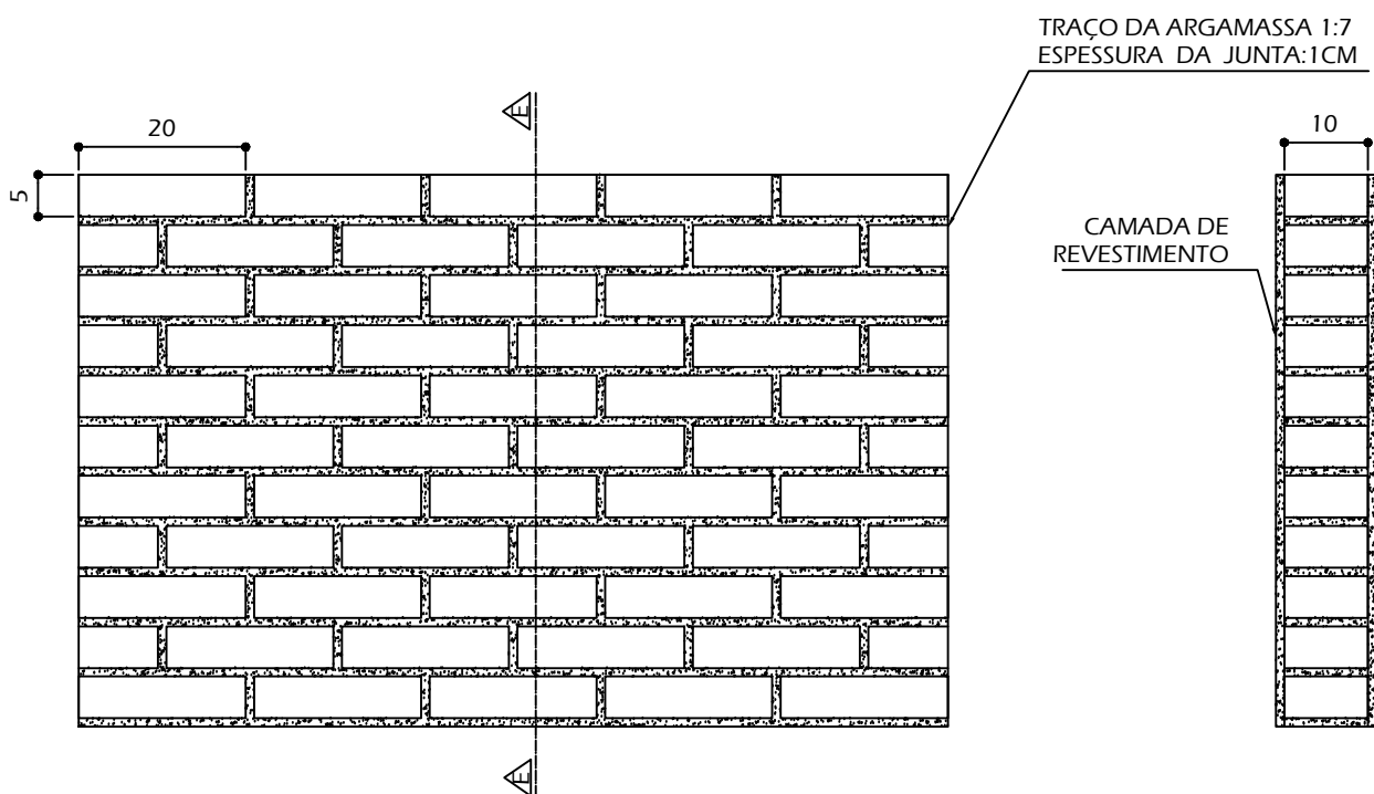
CORTE E-E ESCALA 1/10
