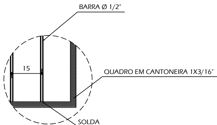
DETALHE 1 ESCALA 1/10
