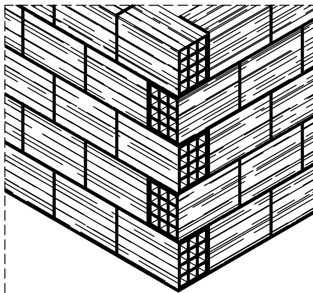
PERSPECTIVA DE AMARRAÇÃO DAS ALVENARIAS
