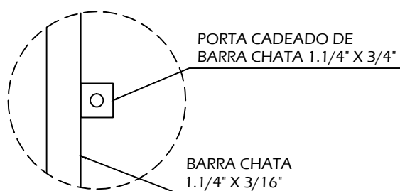
DETALHE 1 ESCALA 1/5
