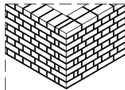
AMARRAÇÃO FRANCESA DE ALVENARIA DE CANTO SEM ESCALA
