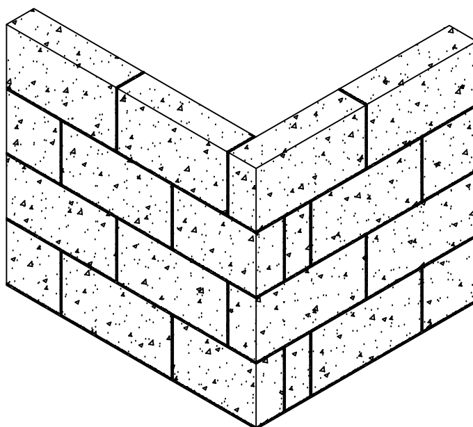
PERSPECTIVA DE AMARRAÇÃO DAS ALVENARIAS SEM ESCALA
