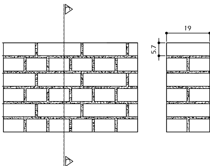
AMARRAÇÃO FRANCESA ELEVÇÃO ESCALA 1/10
