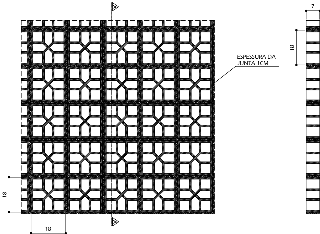
ELEVAÇÃO
