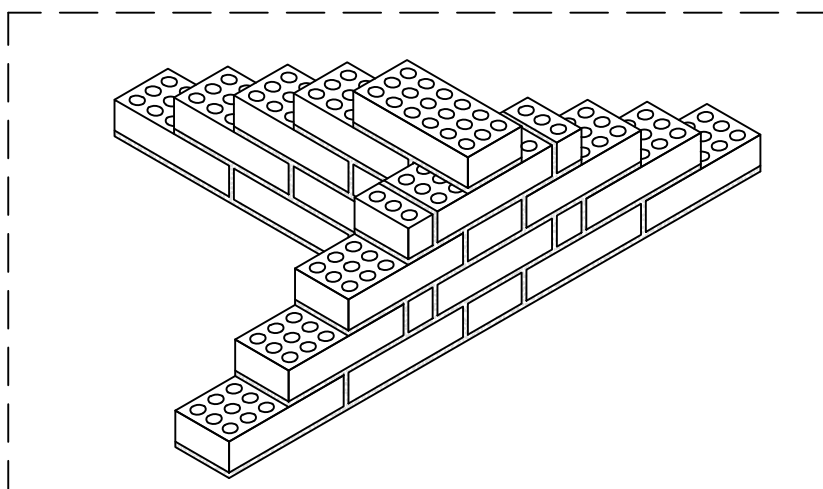
AMARRAÇÃO DE ALVENARIA INTERMEDIÁRIA SEM ESCALA
