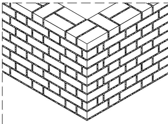
AMARRAÇÃO INGLESA DE ALVENARIA DE CANTO
