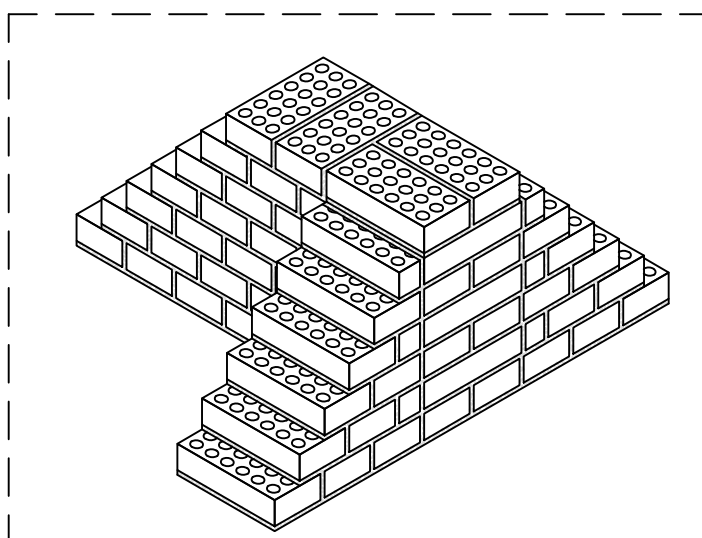
AMARRAÇÃO DE ALVENARIA INTERMEDIÁRIA SEM ESCALA
