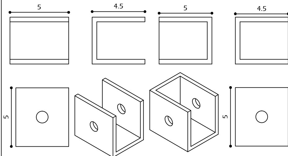
SUPORE PARA UMA PEDRA INTERMEDIÁRIO
