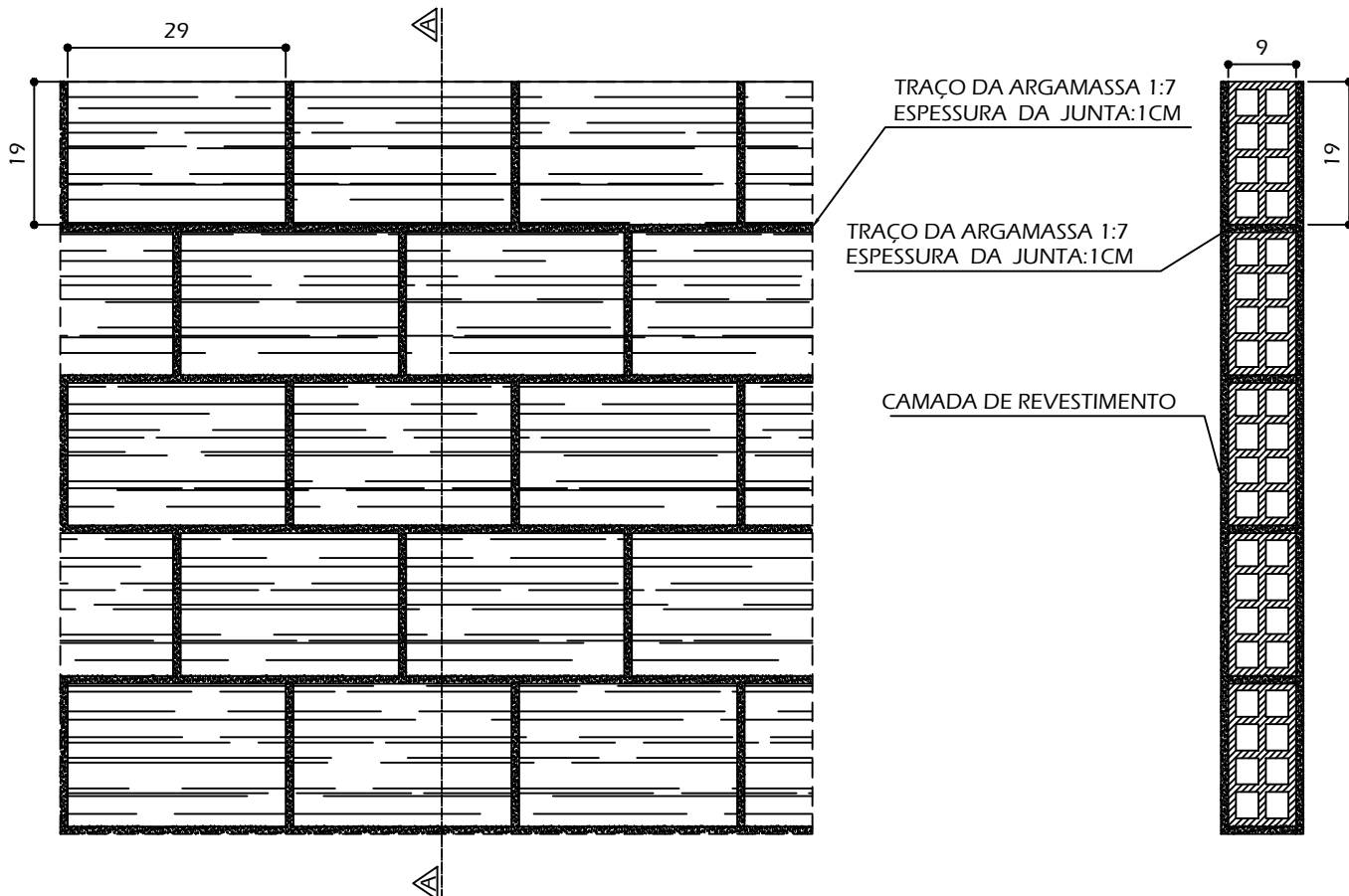
CORTE A-A
