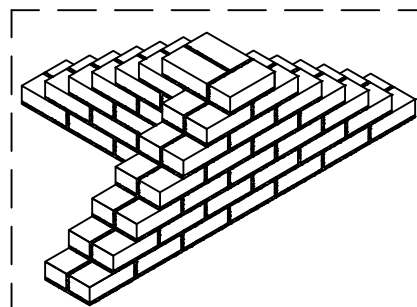
AMARRAÇÃO CONVENCIONAL DE ALVENARIA INTERMEDIÁRIA SEM ESCALA
