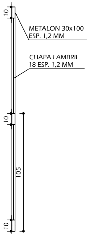
CORTE A-A ESCALA 1/20
