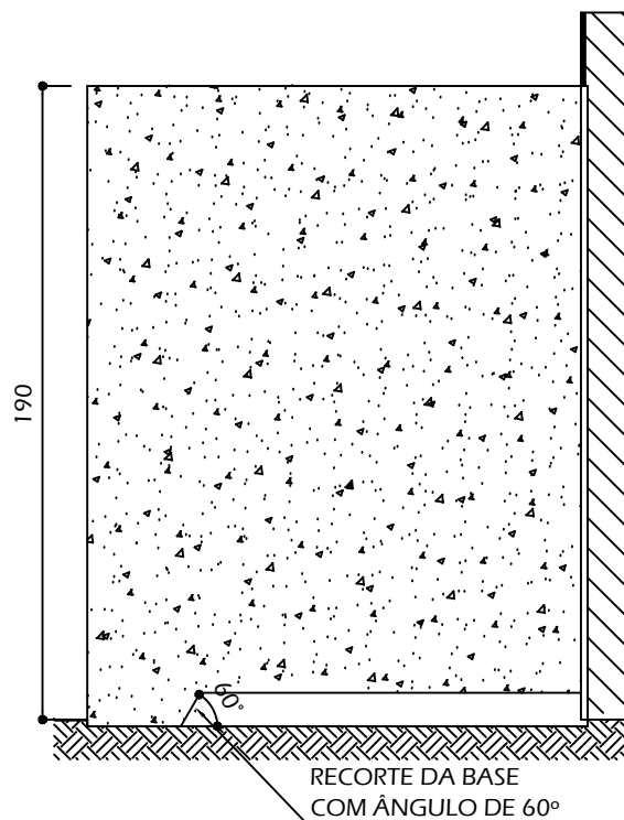
DIVISÓRIA - ELEVÇÃO LATERAL COM RECORTE ESCALA 1/25
