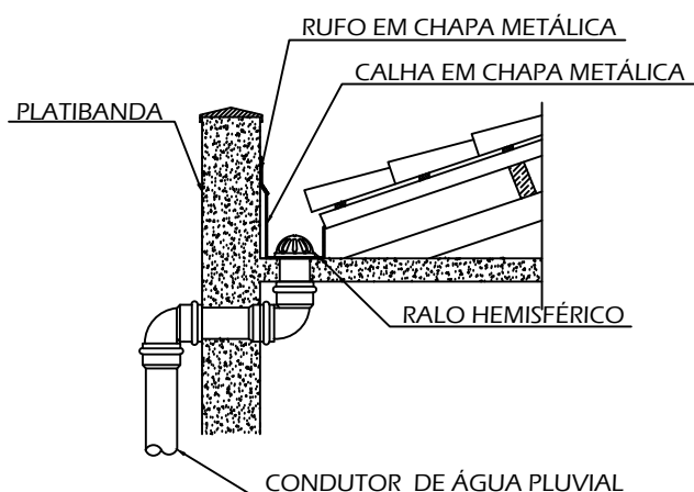
DETALHE 2 - LIGAÇÃO EM TELHADO COM PLATIBANDA SEM ESCALA
