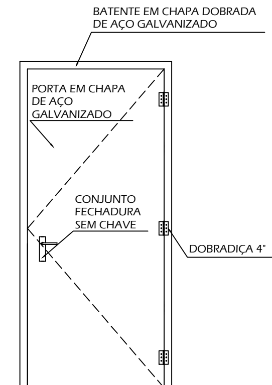
VISTA FRONTAL - PORTA 1 FOLHA
