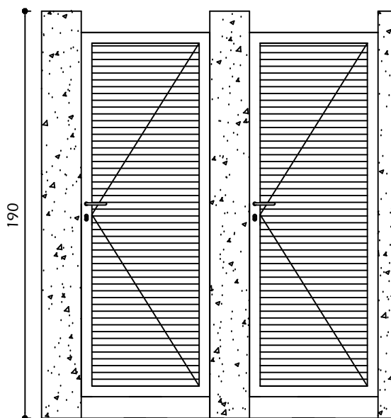
DIVISÓRIA - ELEVACÃO FRONTAL ESCALA 1/25
