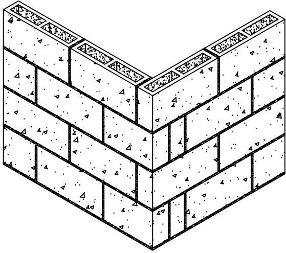
PERSPECTIVA DE AMARRAÇÃO DAS ALVENARIAS
